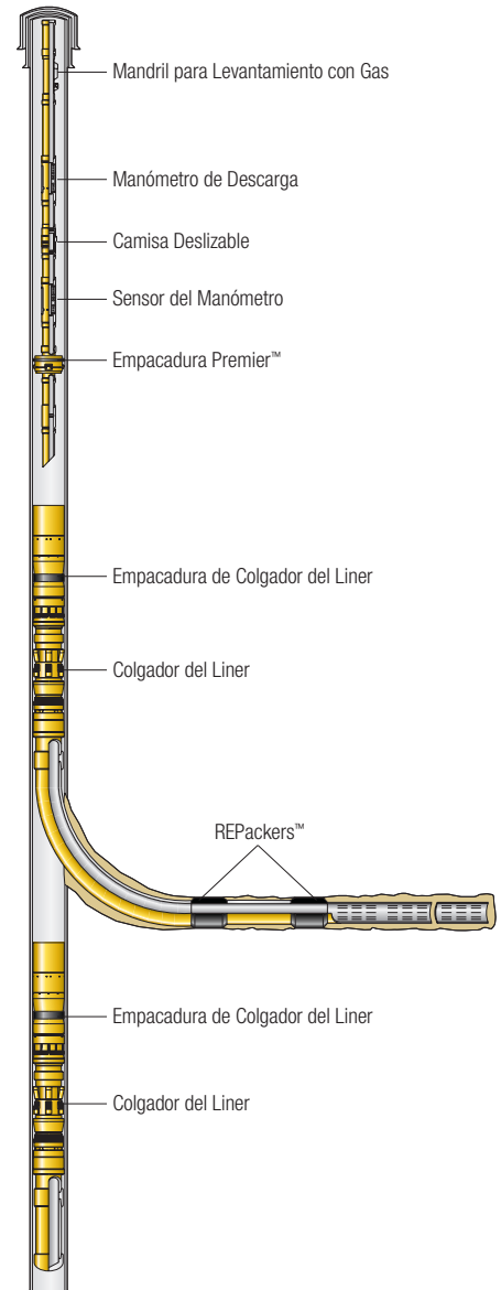
Sistema de empacadura para pozo abierto REPacker™
